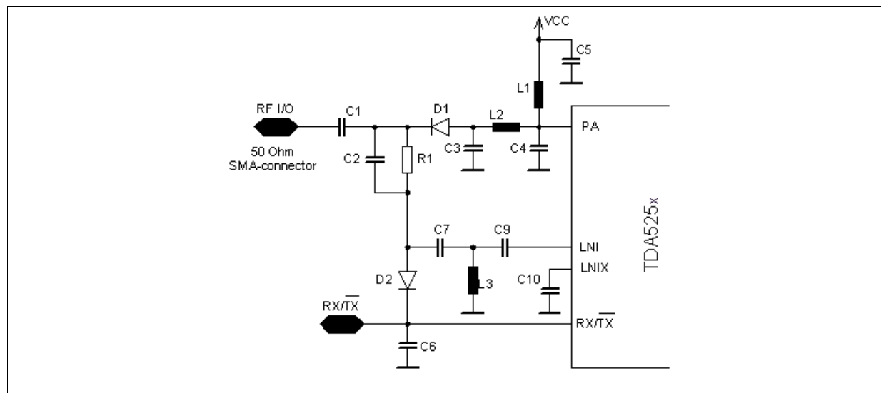
RX/TX_Switch.wmf
